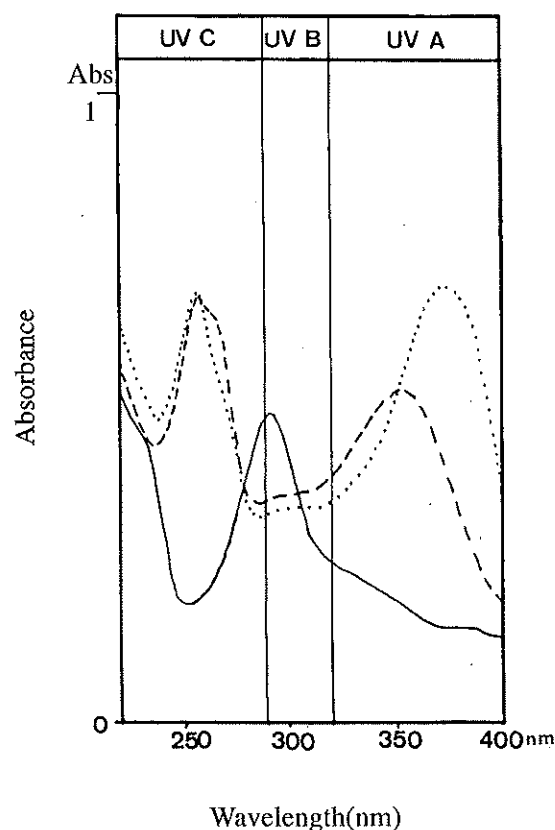
Figure 4. Absorption spectrum of Astilbin (——), Quercetin (.....), Quercitrin (-----).
