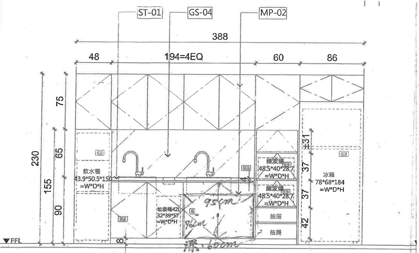
1 茶水間立面圖 SCALE: A3 1/40 A1 1/20
