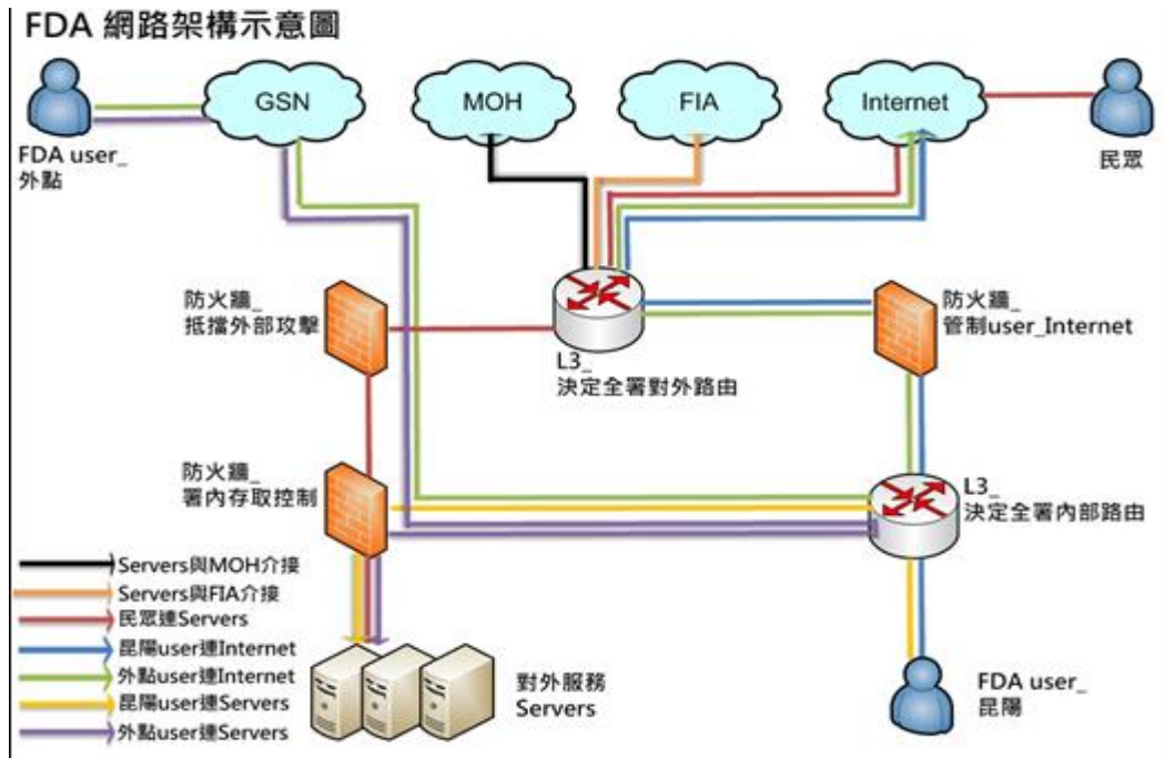
圖 1. 本署網路架構示意圖
