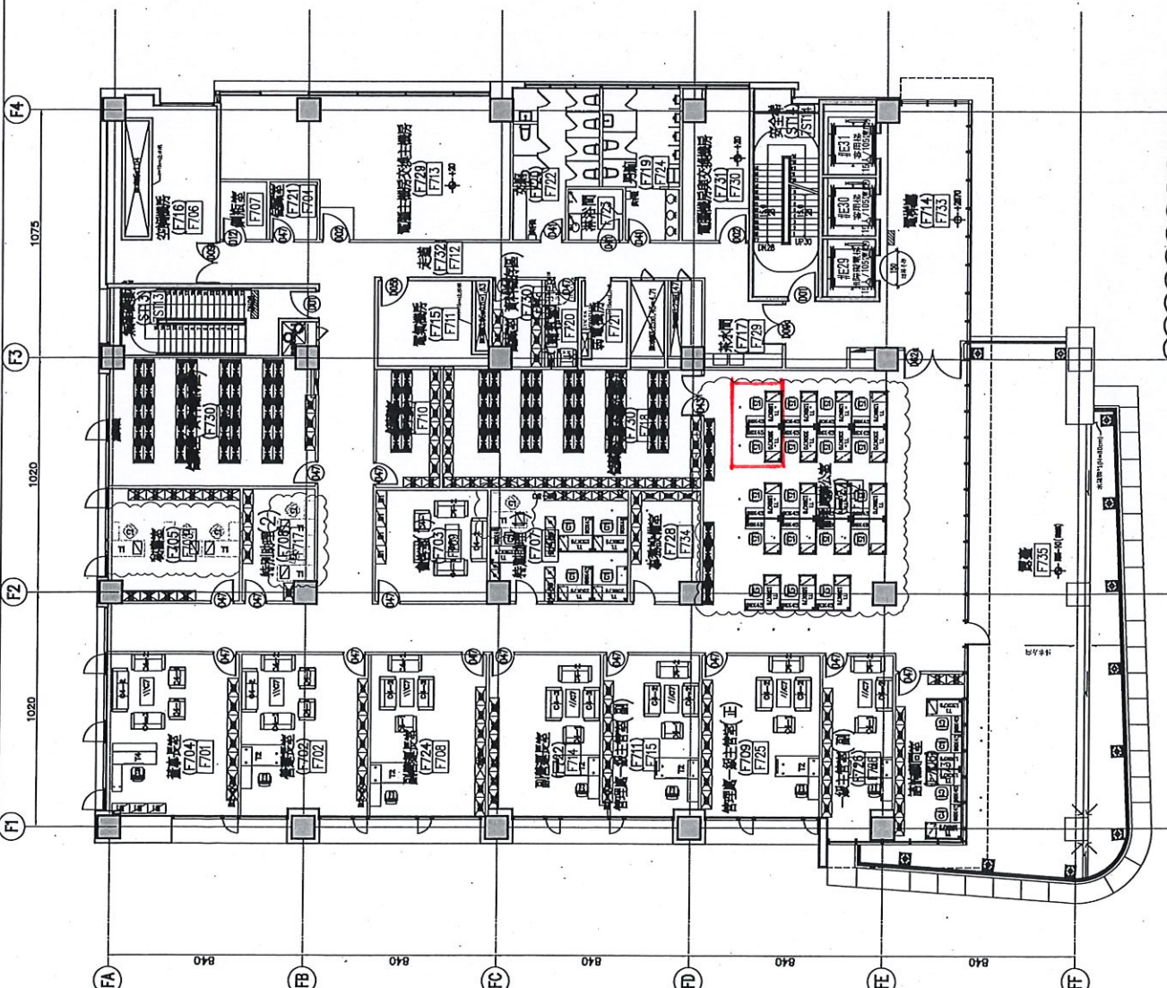
1 煉食品藥物管理署地上七層設備平面圖 A1-S-1/100 A3-S-1/200
